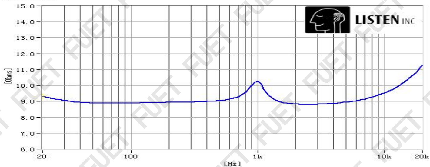
阻抗曲线
