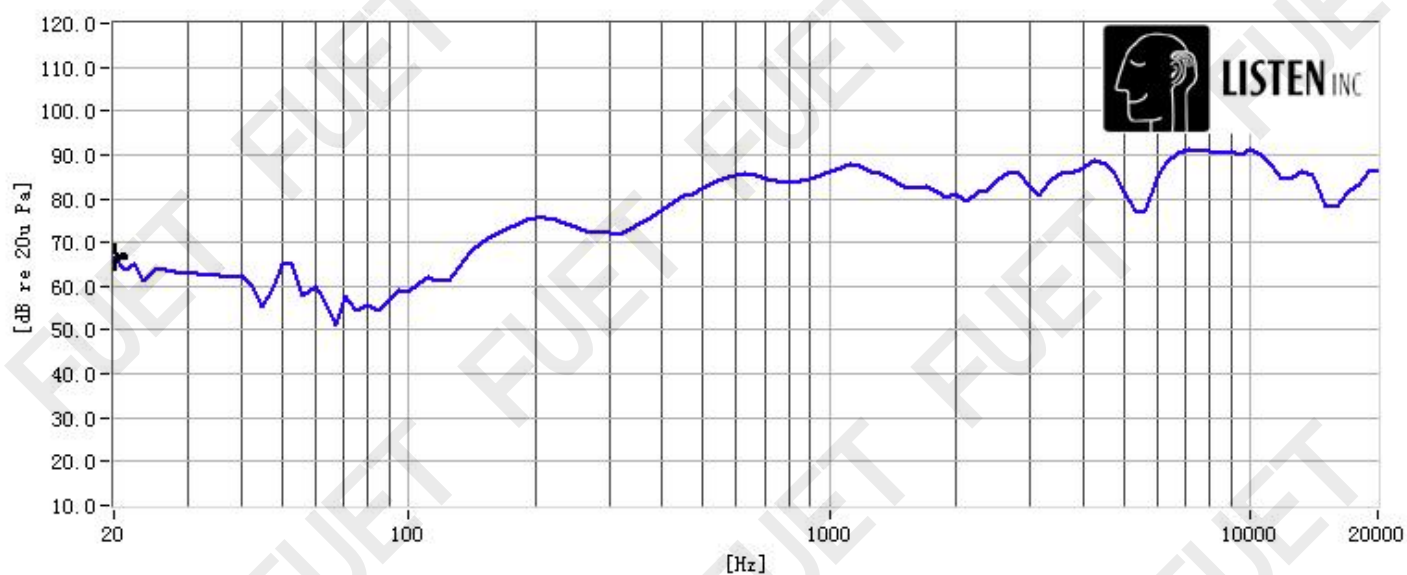
頻响曲线
