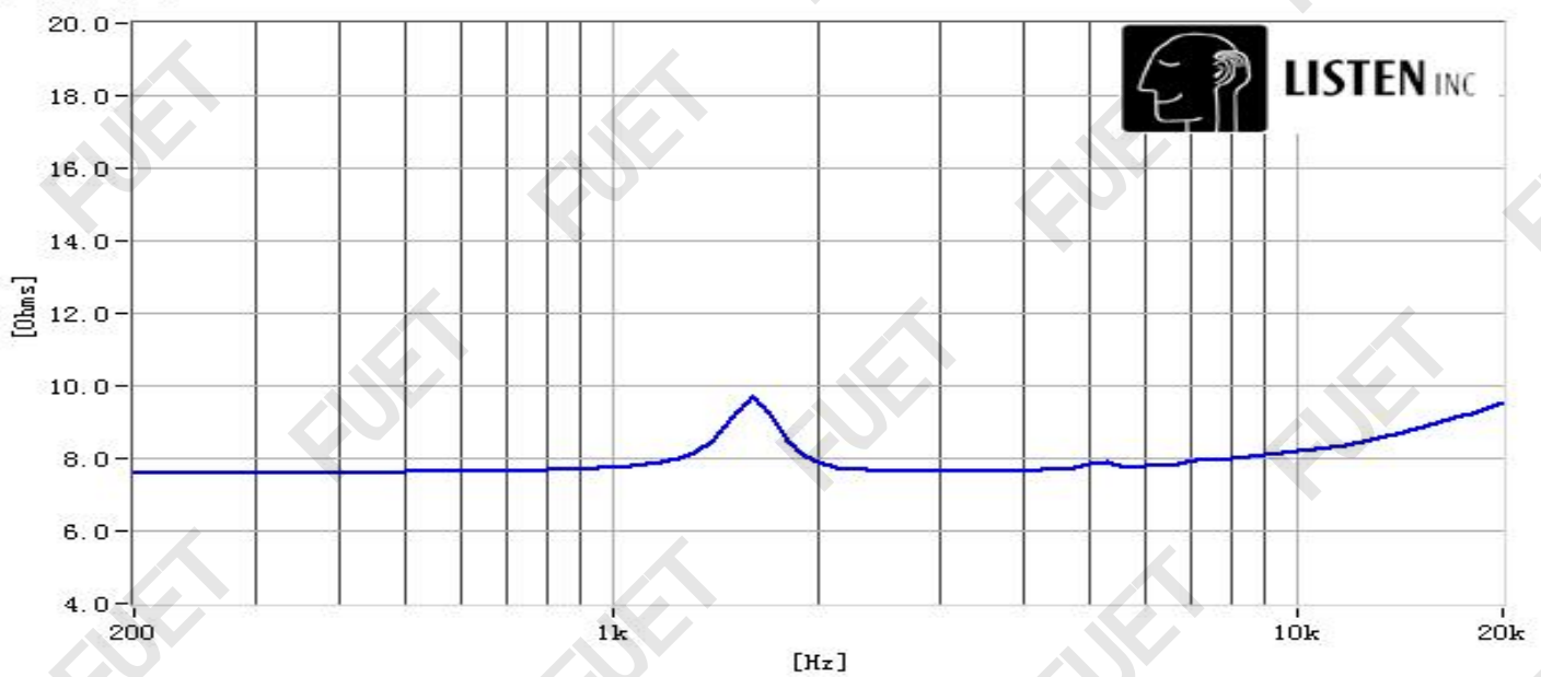
阻抗曲线
